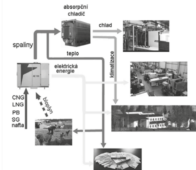
Trigenerace v podmínkách Flídr Využití mikroturbíny pro kombinovanou výrobu tepla a elektrické energie.
